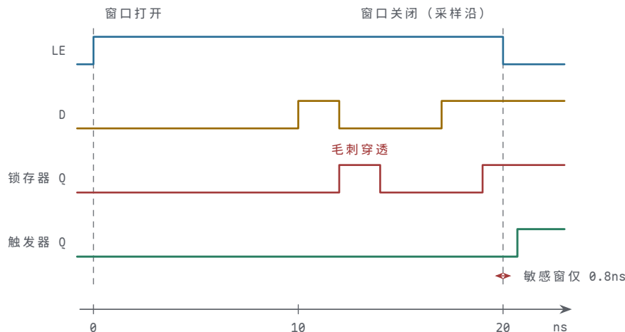
图示：同一个 D 送到两种元件：LE 窗口 ( t=0 到 20\text{ns} ) 内, D 上 2ns 宽的毛刺 ( t=10\text{ns} ) 和晚到的变化 ( t=17\text{ns} ) 都经过约 2ns 延迟穿透到锁存器 Q; D 触发器只认 t=20\text{ns} 采样沿前后共 0.8ns 的窗口, 毛刺完全不可见, 晚到变化被正常采入, 沿后 Q 一步更新。敏感区 20ns 对 0.8ns, 相差 25 倍—这就是透明窗口的代价。
