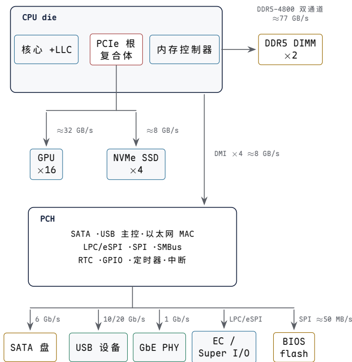
图示：现代 PC 平台拓扑与带宽量级（单向）。CPU die 内的内存控制器与 PCIe 根复合体接管最快的路径：DRAM 直连内存控制器，GPU 与 NVMe SSD 挂在根复合体上；PCH 经 DMI 汇聚全部低速 I/O。注意图上每一处带宽差距都在 10 倍以上—DRAM 约 77 GB/s，DMI 约 8 GB/s，SATA 约 600 MB/s，LPC 与 SPI 只有数十 MB/s—这个落差正是“快
