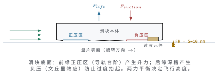
图示：滑块侧视（非等比例）。实际滑块尺寸 \sim 1.25\text{ mm} \times 1.0\text{ mm} ，飞行高度 5-10\text{ nm} ，导轨台阶高度 \sim 50-200\text{ nm} 。
