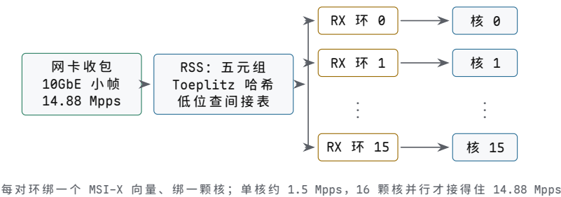
图示：RSS 接收分流：网卡对每帧的五元组算 Toeplitz 哈希，取低位查间接表，把帧定向到对应 RX 环；每对环绑一个 MSI-X 中断向量、绑一颗核，各核独立处理自己环上的帧，提交路径无锁。同一条流哈希相同、永远进同一队列，保序由哈希天然保证；并行度由队列对数决定——10GbE 小帧 14.88 Mpps 对单核约 1.5 Mpps，16 队列绑 16 核才接得住。
