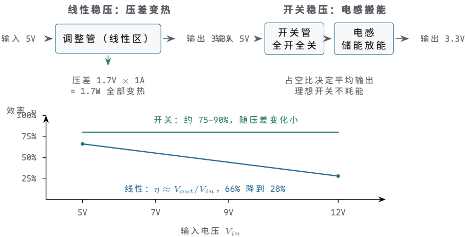
图示：线性稳压与开关稳压的结构对照与效率走势。线性稳压靠调整管串联降压，压差乘电流全部变成热，效率近似等于电压比：5V 转 3.3V 上限 66%，输入换成 12V 只剩约 28%。开关稳压的管子只有全开、全关两个状态，电感在每个周期里储能再放能，把能量一批批搬到输出端，效率约 75%~90%，几乎不随压差改变。压差越大，两条曲线分得越开。
