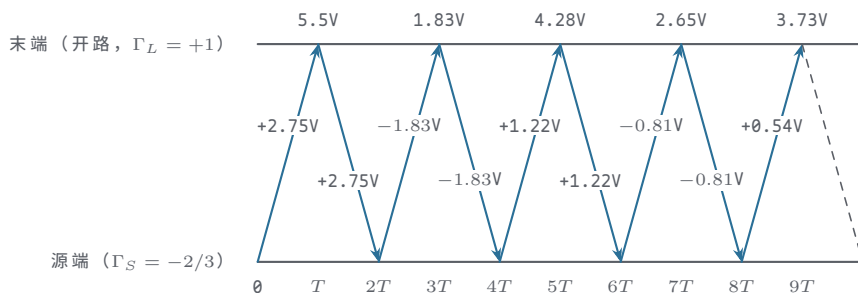
图示：弹跳图：横轴时间、纵轴位置，斜线是行波在源端与末端之间的来回，每跨一次耗时 T 。入射 +2.75\text{V} 在 t=T 到达开路末端， \Gamma_L = +1 全反射，末端跳到 5.5\text{V} ；回波在源端按 \Gamma_S = -2/3 反号弹回，每往返一圈幅度乘 2/3 。上轨标出的各时刻末端电压 5.5 、 1.83 、 4.28 、 2.65 、 3.73\text{V} 与上表逐项一致，逐拍收敛到稳态 3.3\text{V} 。
