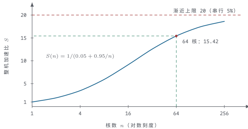
图 12-1 串行占比 5% 时整机加速比随核数的曲线（横轴对数刻度）：8 核 5.93、16 核 9.14、64 核 15.42，之后核数每翻一番，增量越缩越小。红色虚线是 n \rightarrow \infty 的渐近上限 20——串行部分像地板一样等在那里，核数再多也只是无限贴近，永远穿不过去。
