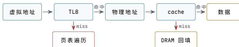
图示：TLB miss 需要地址转换证据；cache miss 需要数据回填证据。二者都可能让 LOAD 变慢，但失败位置不同。
