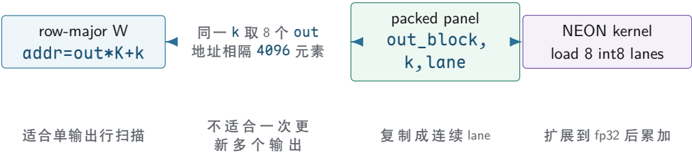
图示：本图要证明的命题是：当前 packed int8 的直接收益是把跨步多输出读取变成连续 lane 读取。
