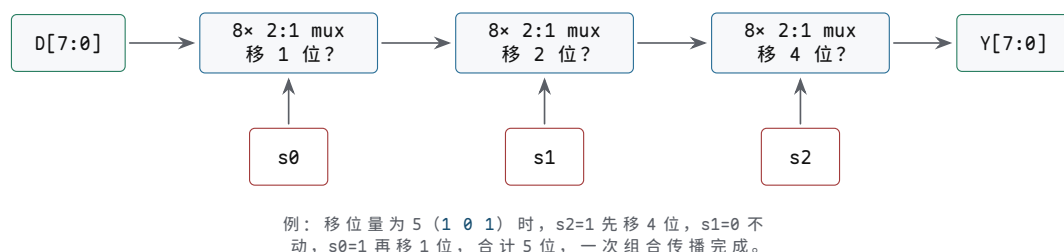
图示：8-bit 桶形移位器：三层 mux 分别由移位量的三个 bit 控制，每一层选择“直送”或“移 2^k 位”。任意 0~7 位移位量都能在一个组合路径内完成，代价是三层 mux 的延迟和大量交叉连线。
