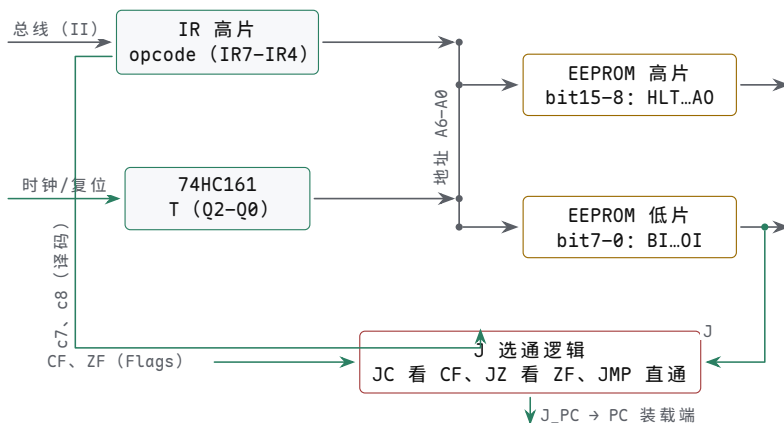
图示：控制单元。IR 高片的 opcode (4 位) 与 74HC161 的 T 状态 (Q2-Q0, 3 位) 拼成 7 位地址，并联送到两片 EEPROM，每片出 8 位，合起来正好 16 根控制线；地址 = opcode×8+T，每条指令占连续 8 行。J 是唯一的例外：它出 ROM 后还要过一级选通——c7、c8 由 opcode 译出，JC 时看 CF、JZ 时看 ZF、JMP 时直通——选通是纯组合逻辑，控制字整拍稳定，拍末采到的是确定电平。
