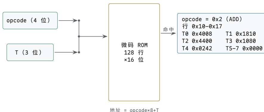
图示：微码查找。7 位地址由高 4 位 opcode 与低 3 位 T 拼成 (地址 = opcode×8+T)，每条指令占据 ROM 中连续 8 行：第 0、1 行是所有指令相同的取指 (C0+MI、R0+II+CE)，第 2 行起按指令分化，用不满的行填 0x0000。图中展开 ADD (opcode 0x2) 的 8 行：T2 送操作数地址、T3 操作数进 B、T4 求和写 A 并记标志，其余三行空转。
