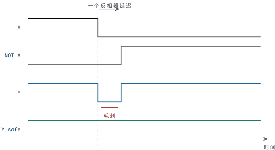
图示： B=C=1 时， Y 的稳定值本应从 1 到 1 不变。但 A 翻转到 NOT A 生效之间隔着一个反相器延迟：上路先关、下路未开， Y 出现一个真值表看不见的窄 0 脉冲。加入共识项 B AND C 后 ( Y_{\text{safe}} )，有一条不依赖 A 的路径全程把输出钉在 1。
