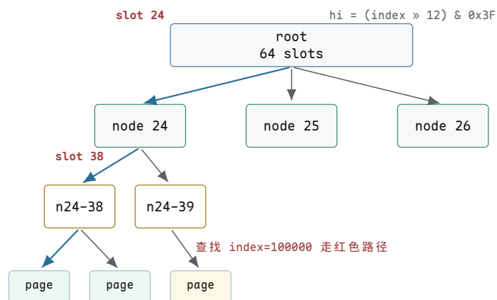
图示：XArray 查找路径。这个教学参数下需要 3 级节点；树高随可表示的索引范围缓慢增长，因此应写成低树高的对数查找，而不是严格 O(1) 。
