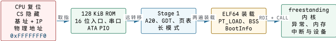
图示：案例的主控制权链。每个阶段都要定义入口处理器状态、可使用的内存、失败后的停机语义和下一阶段入口；缺少任一项，后续成功只能算偶然现象。
