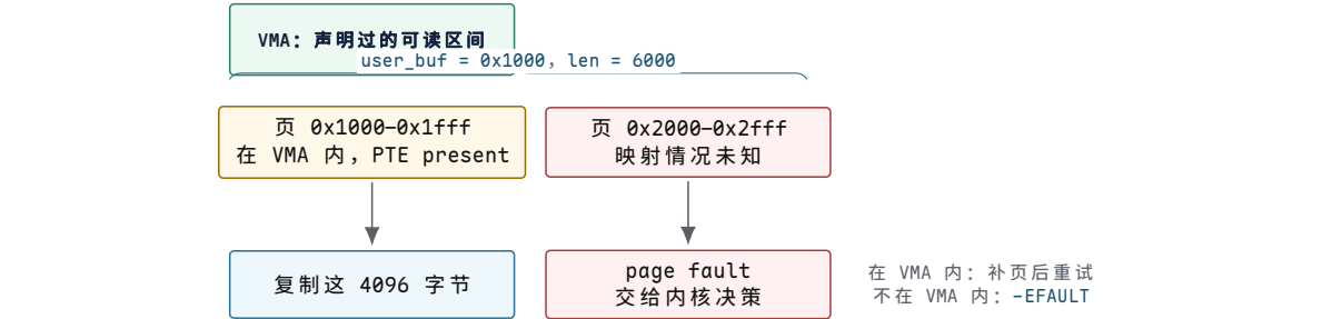
图示：起点 0x1000 合法，只说明第一页可验证；buffer 是一个范围，检查必须按页推进到 0x276f 为止。第二页落入两种结局之一：合法但未装入（补页重试），或根本不属于任何 VMA（拒绝）。
