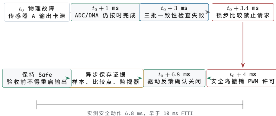
图示：一次传感器卡滞的完整安全时间线。DMA 完成只证明转换结果进入内存；三批一致性窗口确认信息失效，锁步核心产生禁止请求，安全岛撤销独立硬件许可，执行器反馈才确认安全动作完成。证据保存位于关断之后的异步路径，不占用关键 FTTI。
