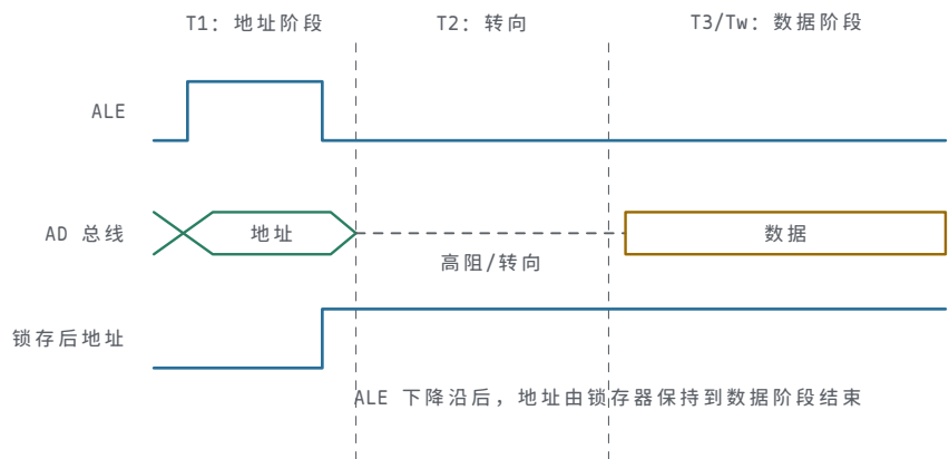
图示：8086 复用总线的读周期：T1 时 ALE 打开锁存窗口，地址随 AD 总线进入锁存器；ALE 落下后窗口关闭，AD 总线转向传数据，而锁存器把地址保持到 T3 采样完成。锁存器把一个总线相位的值变成后续相位仍然可用的状态。
