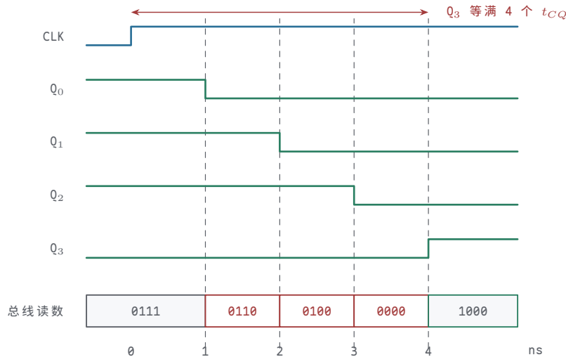
图示：4-bit 纹波计数器从 0111 计到 1000（每级 t_{CQ} = 1\text{ns} ）：CLK 沿后 1ns Q_0 先翻成 0，它的变化再触发 Q_1 ，逐级传递到 Q_3 ，已是沿后 4ns。底部总线行依次读出 0111、0110、0100、0000、1000——红色三格是计数序列中不存在的中问值，后级译码逻辑在这个窗口读数就会看到幻影。同步计数器所有位共享时钟，沿后一步整体更新，没有这些格子。
