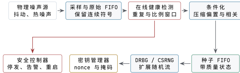
图示：随机数通路两个完成域。健康检测通过只说明当前窗口未观察到规定异常；种子还要经过条件化并带质量状态进入 DRBG。健康检测失败时，控制器停止向密钥消费者提供新熵，而不是继续输出看似随机的数据。
