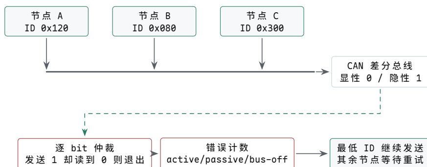
图示：CAN 仲裁与错误隔离共享同一物理反馈：节点边发送边读取总线。仲裁阶段，读到更强的显性 0 表示自己失去优先级但不算错误；数据阶段，发送值与读回值不符合会进入错误计数。协议根据当前阶段解释同一电气事实。
