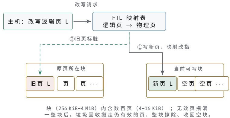
图示：NAND 闪存的页写块擦与 FTL 地址映射。主机以为自己原地改写了逻辑页 L；盘内实际是两步：FTL 把数据写进当前可写块的下一个空页、映射改指新页，旧页标脏等待回收。无效页攒满一整块后，垃圾回收搬走仍有效的页、整块擦除、收回空块—追加写加周期性回收，就是 SSD 在只许追加的介质上提供原地改写接口的全部机制。
