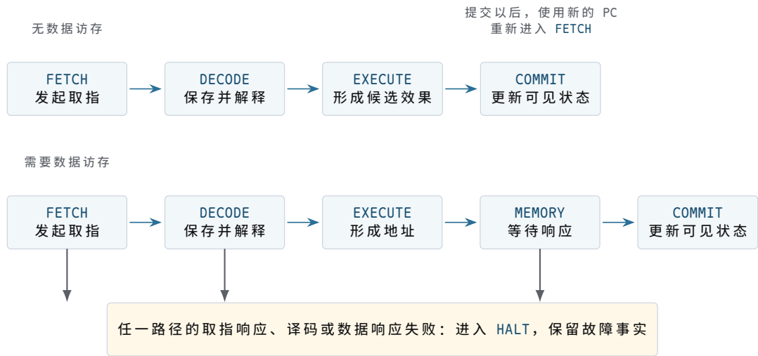
图示：图中一次只有一条指令占据这些阶段。后续若讨论流水线，必须允许许多条指令同时处于不同阶段，并重新定义提交顺序；第一章不预设该结构。
