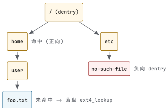
图示：dcache 树：正向 dentry 缓存存在路径，负向 dentry 缓存“不存在”。
