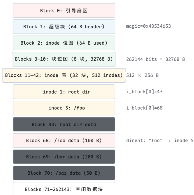
MDFS 磁盘布局 (1 GiB, 262144 块)
