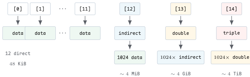
i_block[15] 指针结构
