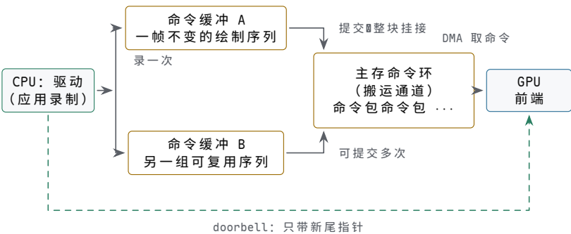
图示：命令缓冲与命令环的二级结构。应用先把命令录进命令缓冲这种可整块复用的对象（录一次），提交时再把整块挂到主存命令环上——一帧里不变的绘制序列录一次、提交多次，驱动省掉重新编码的开销。环只是搬运通道：doorbell 照样只带新尾指针，GPU 前端经 DMA 取命令。构造的成本与提交的成本分开，贵的只做一次，与存储与设备事务相关章节“描述符预先建好、传输时只改指针”是同一招。
