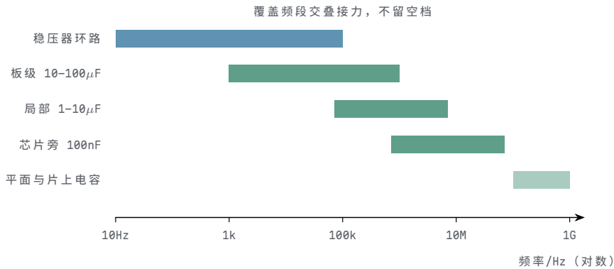
图示：去耦网络按时间尺度分层。储能自上而下逐层减小、响应逐层变快：每层只管自己来得及管的事件，耗尽之前由下一层补仓，最慢的部分留给稳压器环路。
