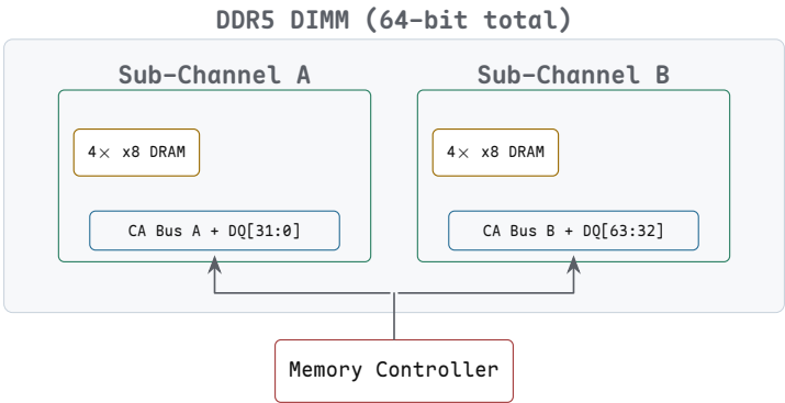
两个子通道完全独立: 可以同时给 A 发 ACTIVATE、对 B 发 READ。每个子通道 32-bit DQ, BL16 仍输出 64 字节 (一条 cache line)。
