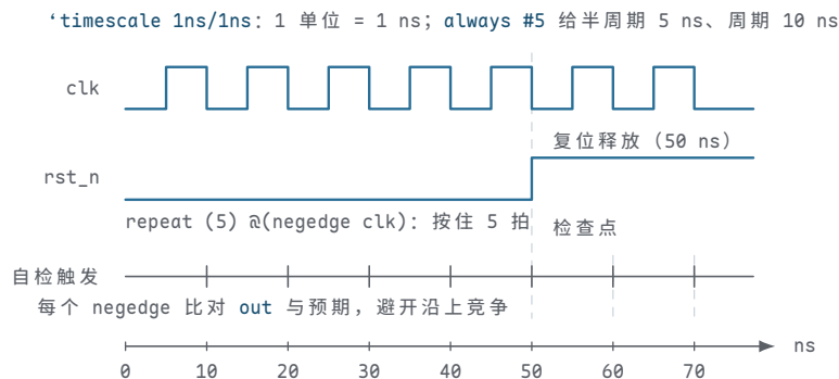
图示：仿真时间轴与三段代码的对应： 'timescale 1ns/1ns 把 1 个时间单位定为 1 ns， always #5 产生周期 10 ns 的时钟；复位拉低后经 repeat (5) @(negedge clk) 按住 5 拍，在第 5 个下降沿（50 ns）释放——刻意选在低电平期间，远离采样沿；自检块在每个下降沿比对 out 与预期，同样避开沿上的读写竞争。RTL 仿真里时间是离散的，这条轴上的每一格都是事件队列里的一个时刻。
