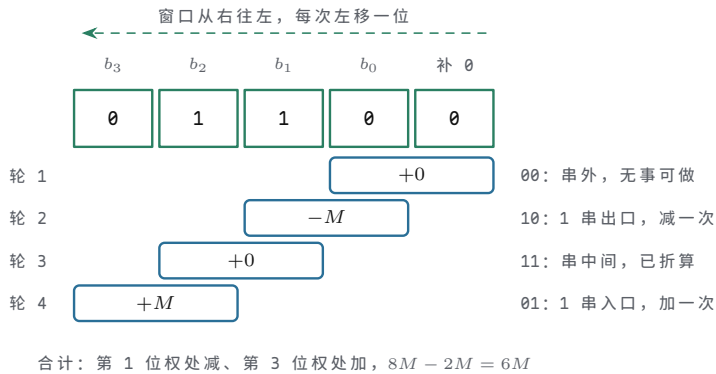
图示：两位 Booth 编码的滑动窗口（乘数 0110，右侧补虚拟 0）。窗口每次只看相邻两位 b_i b_{i-1} ：0→1 是 1 串的入口，对应 +M ；1→0 是出口，对应 -M ；00 与 11 都在串的内部或串外，不累加。四轮中只有轮 2、轮 4 有动作，合计 +M \cdot 2^3 - M \cdot 2^1 = 8M - 2M = 6M ，与乘数值 6 一致——连串 1 被折算成串尾之后的一次减和串首的一次加。
