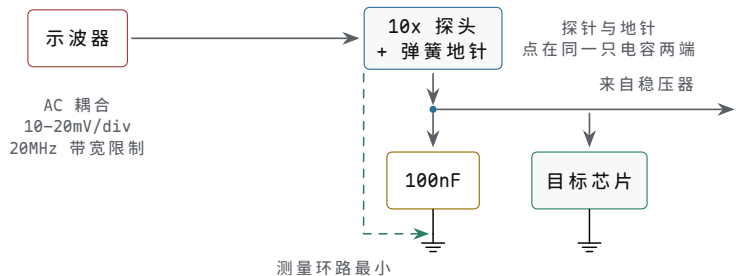
图示：纹波测量的标准接法。示波器切 AC 耦合挡住直流分量，用 10-20mV/div 的档位把纹波展开；10x 探头配弹簧地针，探针与地针直接点在目标芯片电源脚旁那只去耦电容的两端—测的是负载端真实看到的电源，探头围出的测量环路也最小；示波器若有 20MHz 带宽限制就打开，挡住与电源无关的高频拾取。
