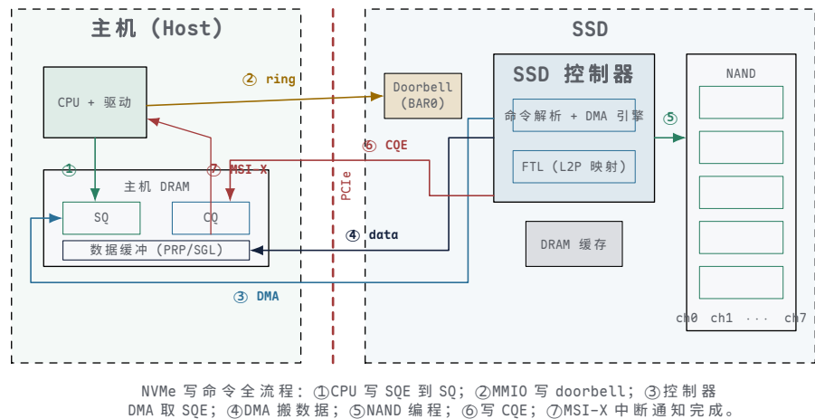
图示：NVMe 命令处理流程。64K 队列 × 64K 深度允许数万条命令同时在途（in-flight），远超 AHCI 的单队列 32 深度。多队列可绑定到不同 CPU 核，消除锁竞争。
