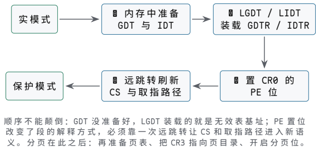
图示：从实模式进入保护模式的硬件步骤链（80386）。准备描述符表、装载 GDTR/IDTR、置 CR0 的 PE 位、远跳转刷新取指路径与段状态，四步都是硬件状态切换，顺序错误会让取指、数据访问或异常入口无法解释；若还要分页，需在此之后再准备页目录和页表、装载 CR3、开启分页控制位。
