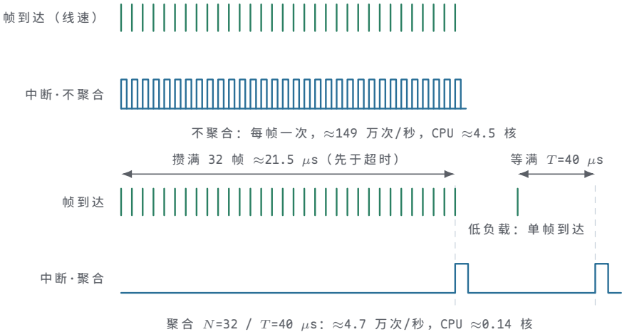
图示：中断聚合的时序对比。上方不聚合：每帧一次中断，1.49 Mpps 折合每秒约 149 万次中断进出，约 4.5 颗核的算力全花在保存与恢复现场上。下方聚合：攒满 32 帧（线速下约 21.5\ \mu\text{s} ，先于超时）或等满 T=40\ \mu\text{s} ——先到为准——才发一次中断，中断率降到约 4.7 万次/秒，CPU 开销约 0.14 核；代价是一帧平均多等约半个聚合窗口。
