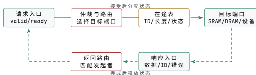
图示：多笔在途事务的状态闭环。请求在握手沿被接受后占用一项在途状态；响应按 ID 返回并累计 beat，只有数据完整或错误被确认后才释放。请求、接受、响应与完成是四个不同边界。
