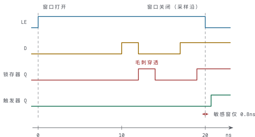
图示：同一个 D 送到两种元件：LE 窗口 ( t=0 到 20\text{ns} ) 内，D 上 2ns 宽的毛刺 ( t=10\text{ns} ) 和晚到的变化 ( t=17\text{ns} ) 都经过约 2ns 延迟穿透到锁存器 Q；D 触发器只认 t=20\text{ns} 采样沿前后共 0.8ns 的窗口，毛刺完全不可见，晚到变化被正常采入，沿后 Q 一步更新。敏感区 20ns 对 0.8ns，相差 25 倍——这就是透明窗口的代价。
