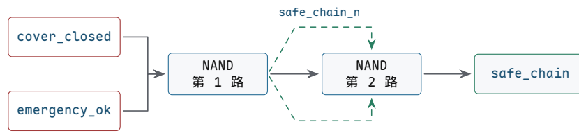
第二路 NAND 的两个输入接同一个反相信号，等价于把第 1 路输出再反相。图中分成两条回入线，是为了避免箭头穿过文字。
