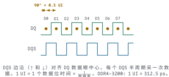
图示：DQS/DQ 对齐关系。DQS 相对 DQ 偏移 90^\circ (即四分之一 DQS 周期，0.5 UI)，使 DQS 的上升沿和下降沿恰好落在 DQ 数据有效窗口的中心。
