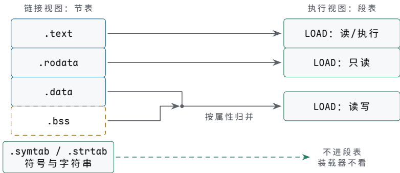
图示：同一份字节的两种看法。链接视图按节组织：名字、类型、大小与属性逐项登记在节表里，链接器按节合并、按节定址；执行视图把属性相同的节归并成 LOAD 段，只保留虚拟地址、文件范围与读写执行权限，装载器只看这一份。可重定位文件通常只有节表；可执行文件两份都有，装载时只用段表——strip 把节表整个剥掉，程序照样运行。
