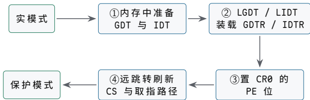
顺序不能颠倒：GDT 没准备好，LGDT 装载的就是无效表基址；PE 置位改变了段的解释方式，必须靠一次远跳转让 CS 和取指路径进入新语义。分页在此之后：再准备页表、把 CR3 指向页目录、开启分页位。
