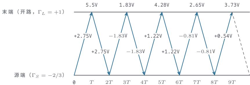
图示：弹跳图：横轴时间、纵轴位置，斜线是行波在源端与末端之间的来回，每跨一次耗时 T 。入射 +2.75V 在 t=T 到达开路末端， \Gamma_L = +1 全反射，末端跳到 5.5V；回波在源端按 \Gamma_S = -2/3 反号弹回，每往返一圈幅度乘 2/3。上轨标出的各时刻末端电压 5.5、1.83、4.28、2.65、3.73V 与上表逐项一致，逐拍收敛到稳态 3.3V。
