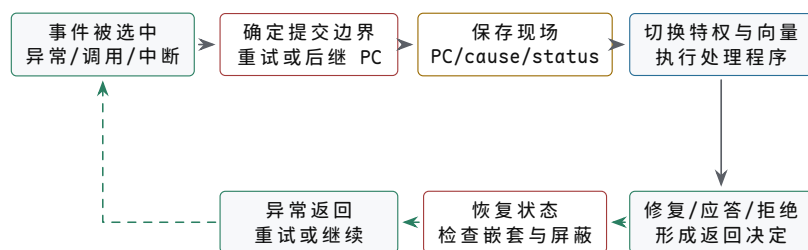
图示：陷阱的闭环由两条路径组成：上排在一个可恢复边界保存架构状态并进入处理程序；下排先消除或确认事件，再恢复状态并选择重试故障指令或从后继 PC 继续。返回指令提交之后，旧特权上下文才重新拥有执行权。
