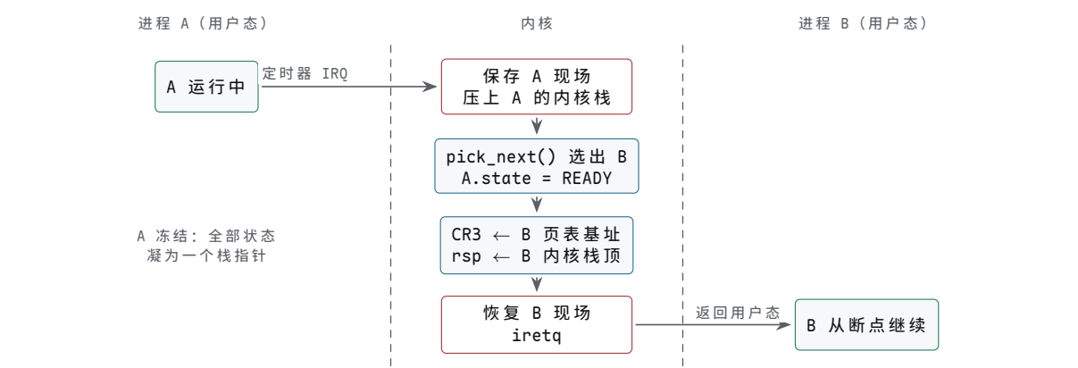
图示：上下文切换泳道（对应正文 trace）。定时器中断在指令边界把 CPU 从 A 带进内核：A 的现场压上它自己的内核栈，调度器选出 B 后写入 B 的页表基址（CR3）、把栈指针切到 B 的内核栈，再弹出 B 的寄存器并 iretq —返回落进 B 的用户态，B 只觉得上次陷入返回得特别久。被切走的 A，全部状态归结为进程控制块里的一个栈指针，等下次被选中时原路恢复。
