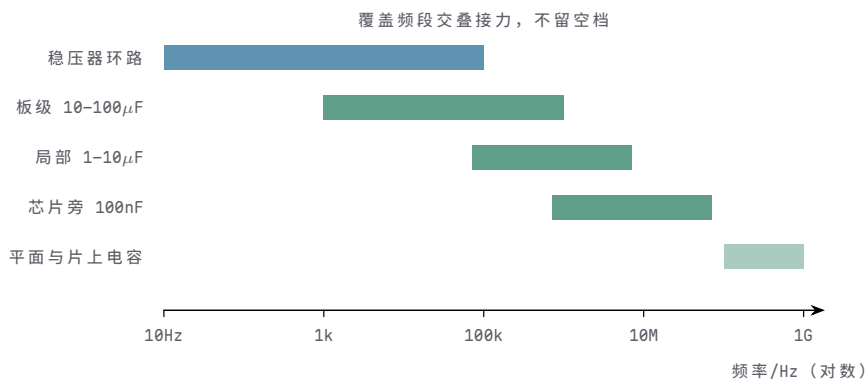
图示：各层电容在频率轴上的分工。稳压器环路管 100kHz 以下的慢变化；板级电解、局部 \mu\text{F} 级、芯片旁 100nF 按各自自谐振频率错开接力—10 \mu\text{F} 自谐振约 0.7MHz，100nF 约 7MHz；100MHz 以上分立电容无能为力，由电源-地平面对的平面电容与片上电容收尾。相邻层的覆盖频段交叠，合成阻抗曲线才不会在任何频段冒过目标线。
