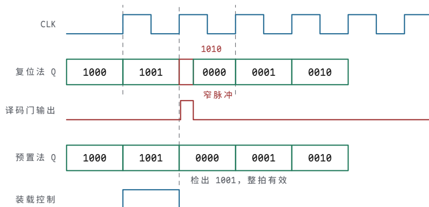
图示：复位法（上）：第 10 个时钟沿后，加一结果 1010 作为瞬态出现几纳秒（红色窄格），译码门检出后输出一条窄清零脉冲把各级拉回 0000——脉冲宽度只有“译码门延迟加清零响应”那么长，各级清零速度不齐时可能清不干净。预置法（下）：译码门在 1001 的整个周期内拉起装载控制，下一个时钟沿把 0000 装入，1010 从头到尾不出现，序列里没有任何瞬态。
