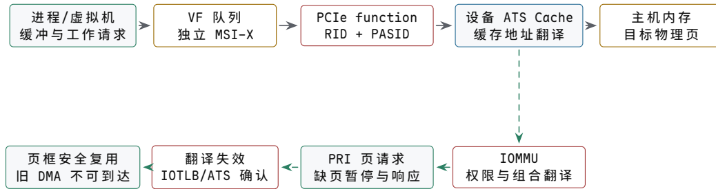
图示：共享设备的一次 DMA 同时携带 function 身份和进程地址空间身份。ATS 允许设备缓存 IOMMU 翻译，PRI 允许缺页时请求软件补页；撤销页面时必须停止新工作并让 IOMMU 与设备翻译缓存都确认失效，旧页框才能复用。
