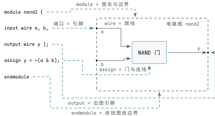
图示：这几行代码与电路图元的逐项对应（虚线为对应关系，不是电路连接）： module/endmodule 圈出图纸边界，端口表给出进出图的三根引脚， wire 是引脚到门之间的跳线， assign 把一只 NAND 门接在 a 、 b 与 y 之间。读任何 module 都用这个顺序：先看引脚，再数跳线，最后对每个门对号入座。
