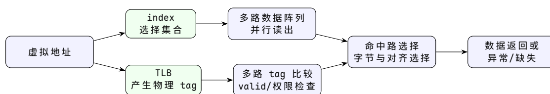
图示：一次 L1 读取的并行关键路径。集合选择与 TLB 翻译同时开始，物理 tag 比较结果再选择对应数据路；图中上下分支之间保留间距，以区分数据阵列和翻译比较两条路径。
