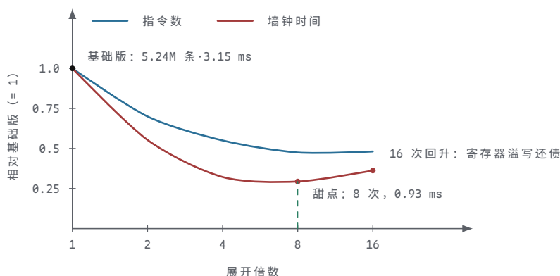
图示：循环展开 1、2、4、8、16 倍的两条归一化曲线（基础版 = 1，对应 5.24M 条指令、3.15 ms）。指令数随展开单调下降——循环开销被摊薄；墙钟时间先降后升，8 次的 0.93 ms 是甜点：8 个累加器加 8 个 load 目标恰好顶到寄存器堆容量。展开 16 次后寄存器不够用，中间值溢写到栈上，指令数与 CPI 双双回升。
