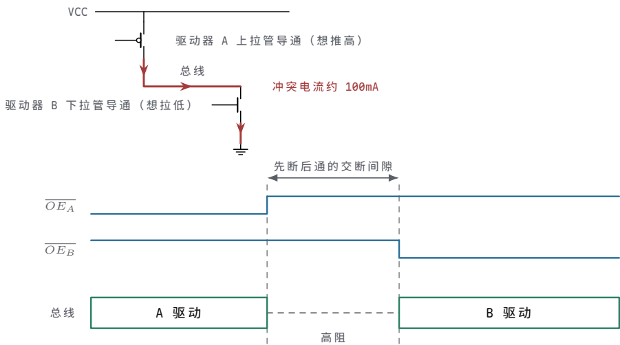
图示：上：两个三态驱动者同时使能时的冲突通路——电流从 VCC 经 A 的上拉管、总线、B 的下拉管直到 GND（图中只画出导通的管子，另一只方向的管子均关断），按每个输出级导通电阻约 25\Omega 估算约 100\text{mA} ，总线电平停在中点附近，既不是合法高也不是合法低。下：正确的驱动权交接——A 的使能先撤、输出进入高阻，留出先断后通的切换间隙后 B 才使能，任何时刻总线上最多一个驱动者。
