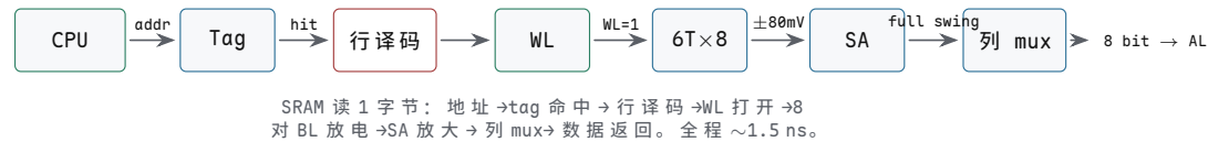
图示：SRAM 读路径。每一步都是组合逻辑或单级放大，没有等待状态，因此 L1 访问可以在一个时钟周期内完成。
