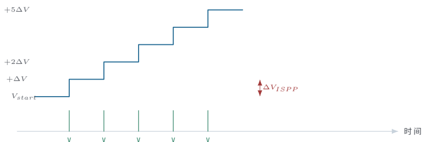
ISPP 阶梯波形：每个编程脉冲后跟一次验证 ( V )。未通过的单元在下一个更高脉冲中继续注入电子。 \Delta V_{ISPP} 典型 0.2\text{--}0.5\text{V} 。
