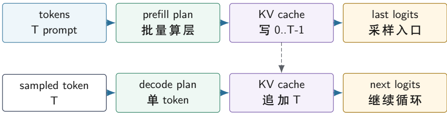
last logits 经 sampler 产生下一行的 decode 输入；prefill 写入的历史在 decode 阶段继续可读，decode 每步再追加一个位置。
