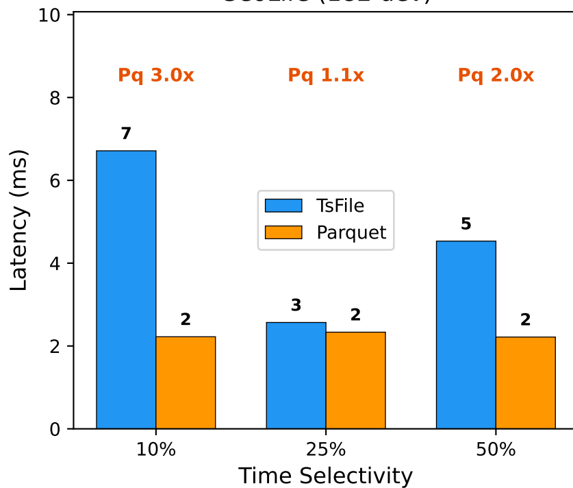
GeoLife (182 dev)
