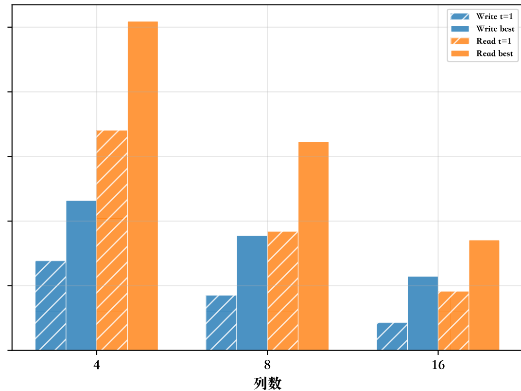
LZ4
