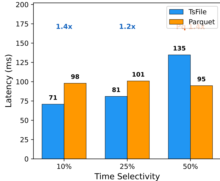
TSBS (100 dev)
