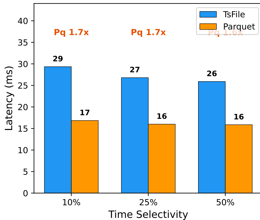
GeoLife (182 dev)
