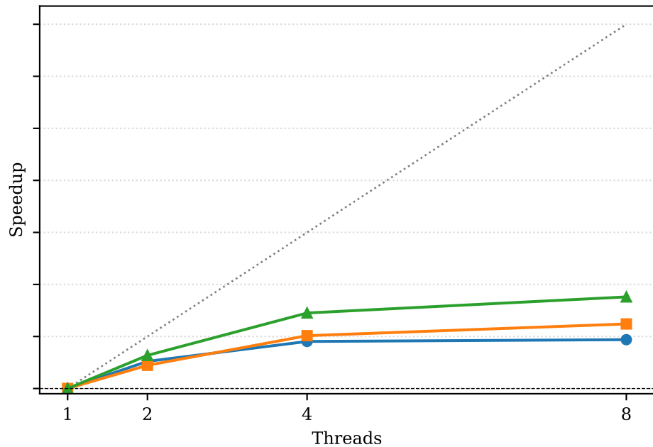
LZ4
