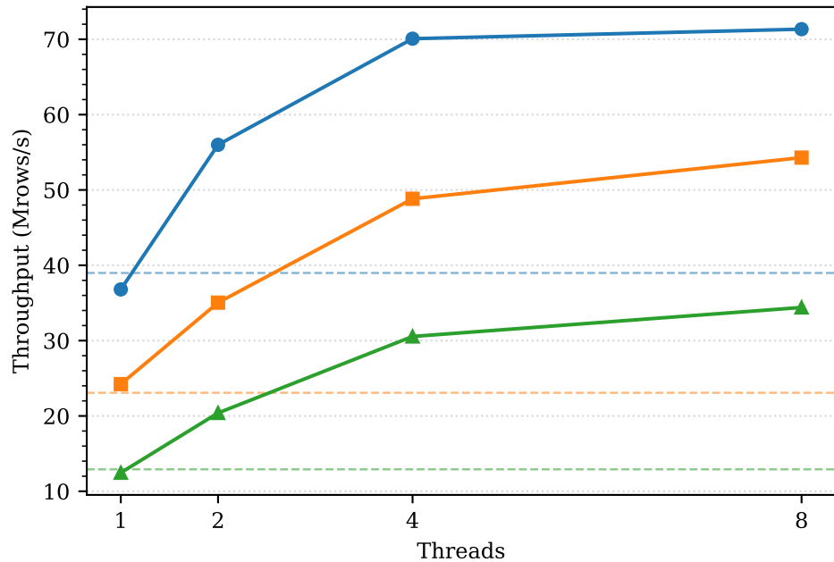
LZ4
