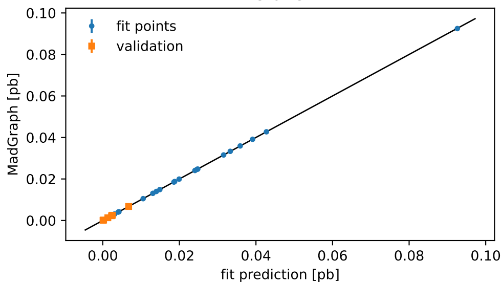
14 TeV
