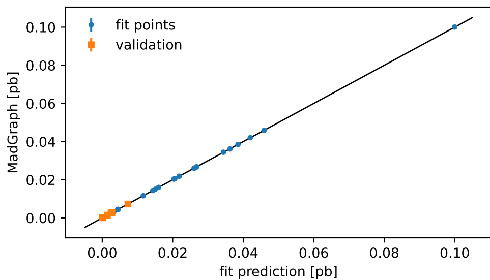
14 TeV
