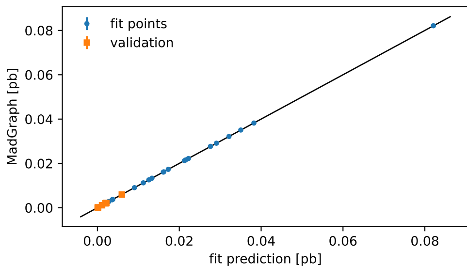
13.6 TeV
