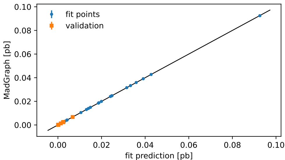
14 TeV
