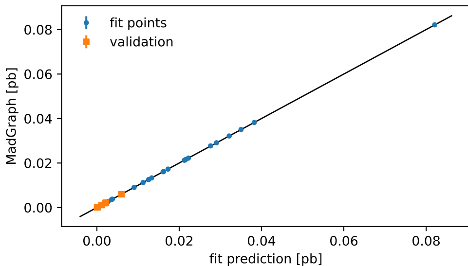
13.6 TeV
