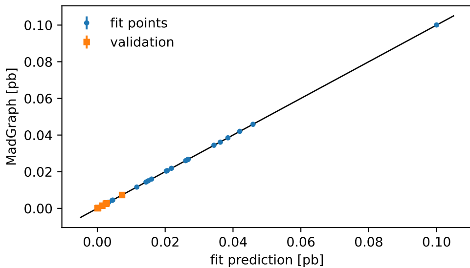
14 TeV
