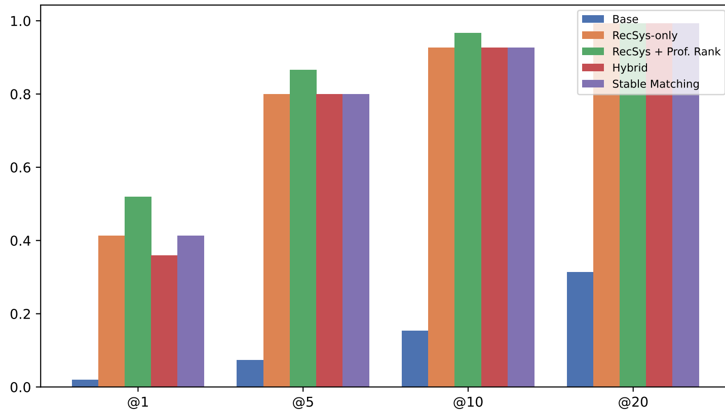
HitRate@K
