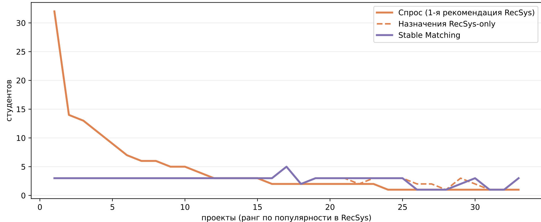
Stable Matching сглаживает перегруз популярных проектов
