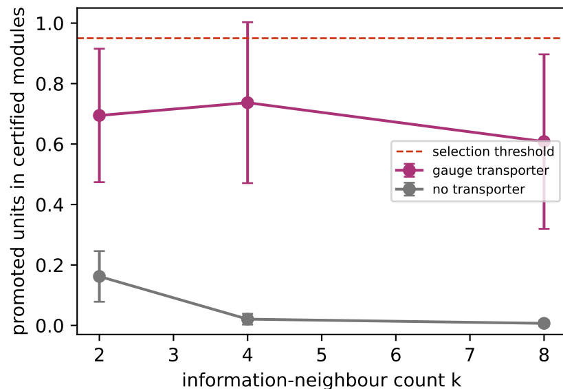
(d) Certification across scale
