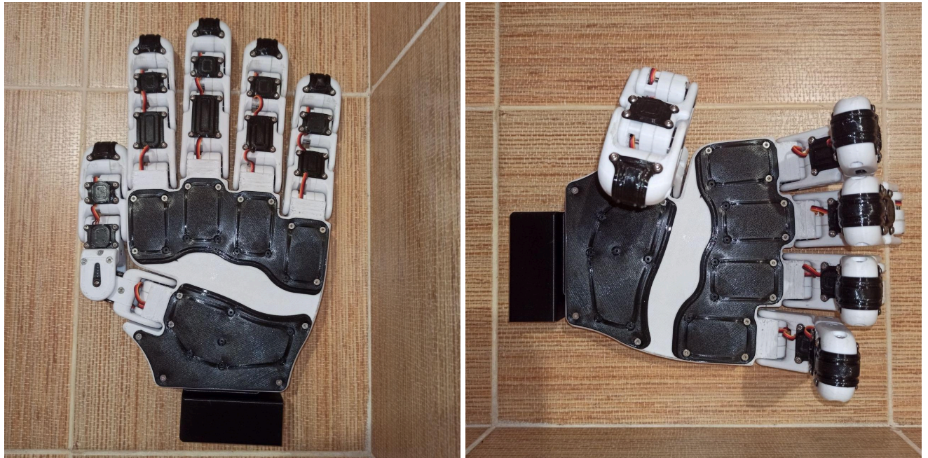
Рисунок 4.2 — Фото готової роботизованої руки
