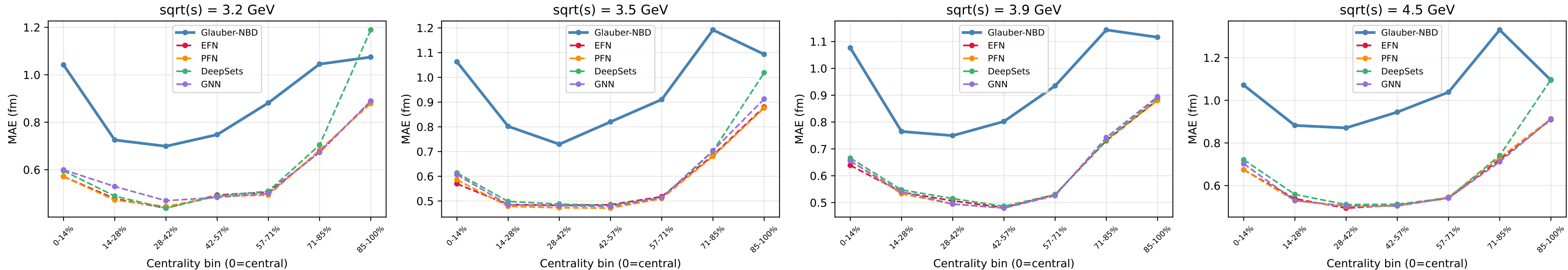
MAE per centrality bin (test set)
