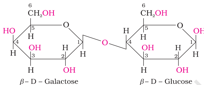
Lactose
