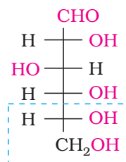
D-(+) - Glucose
