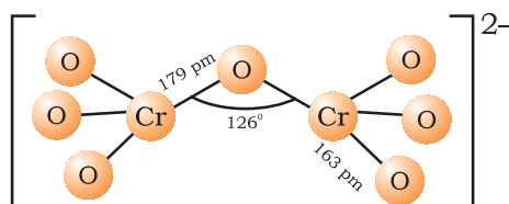
Dichromate ion
