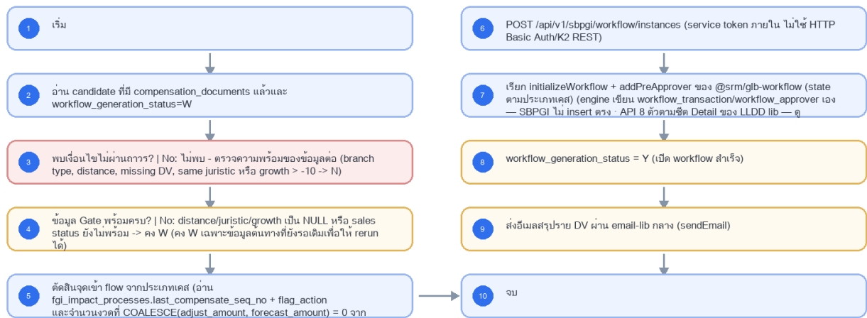
รูปที่ 1: Implementation flow reference: LLDD BE - Job 8b StartInternalWorkflow
