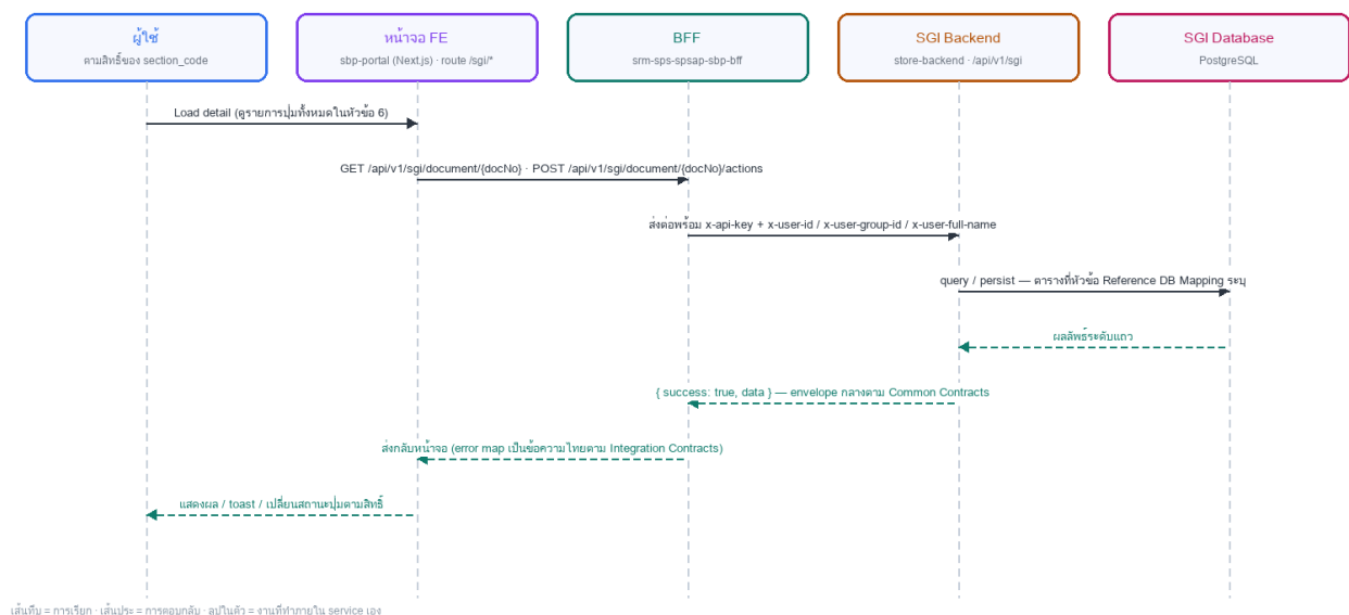
รูปที่ 2: Sequence diagram: LLDD FE - Document Detail Role 01 Business Promotion
