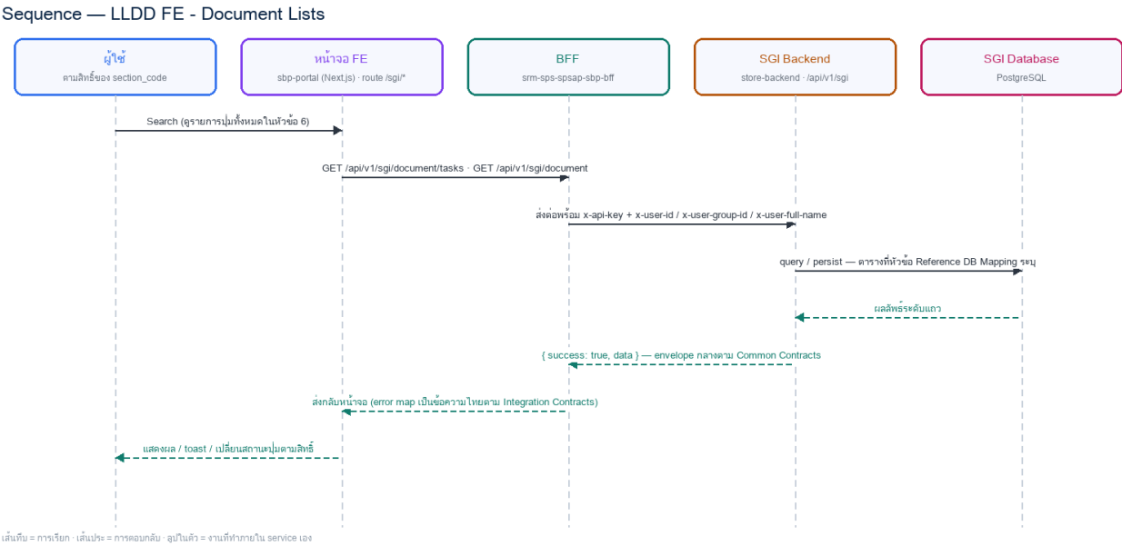
รูปที่ 5: Sequence diagram: LLDD FE - Document Lists
