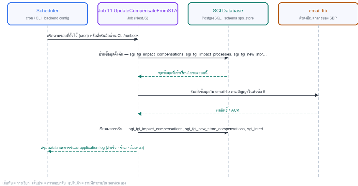
รูปที่ 2: Sequence diagram: LLDD BE - Job 11 UpdateCompensateFromSTA
