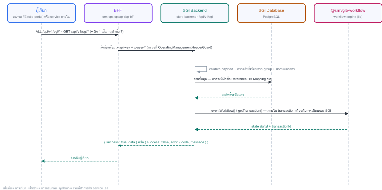
รูปที่ 2: Sequence diagram: LLDD BE - API Common Contracts
