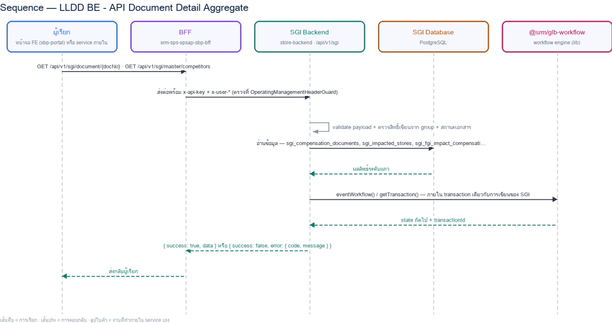
รูปที่ 2: Sequence diagram: LLDD BE - API Document Detail Aggregate
