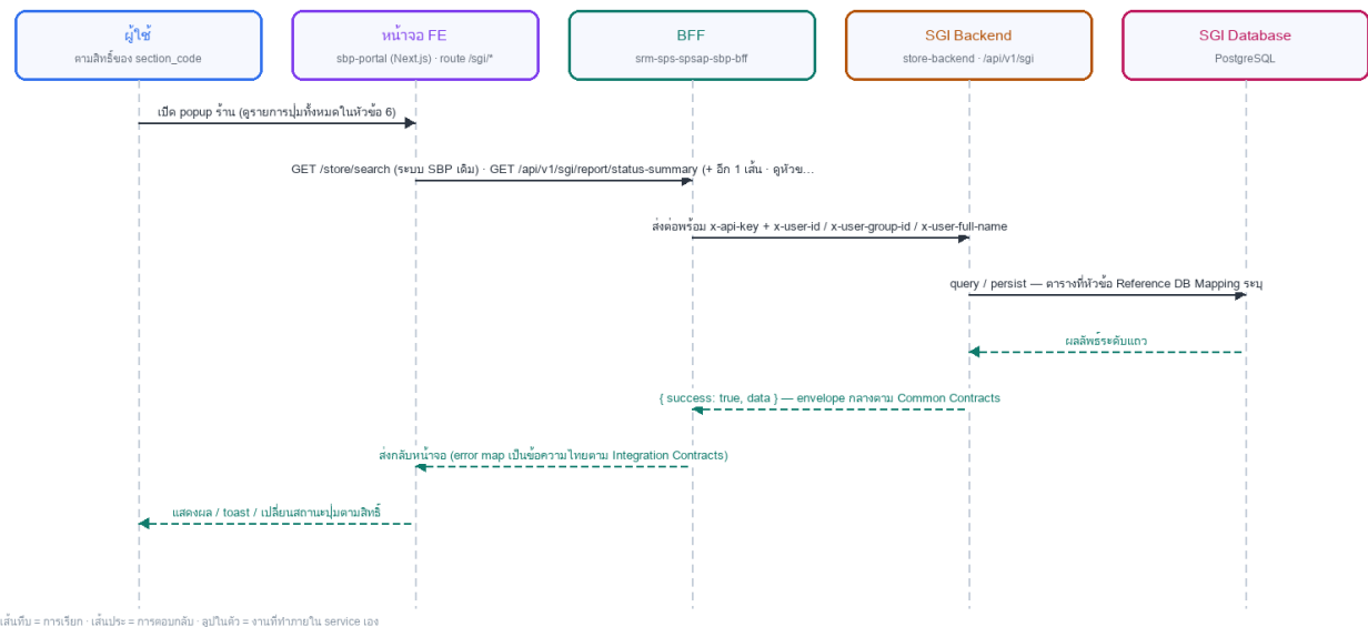
รูปที่ 4: Sequence diagram: LLDD FE - Status Summary Report
