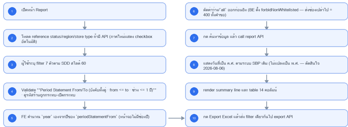
รูปที่ 3: Implementation flow reference: LLDD FE - Status Summary Report
