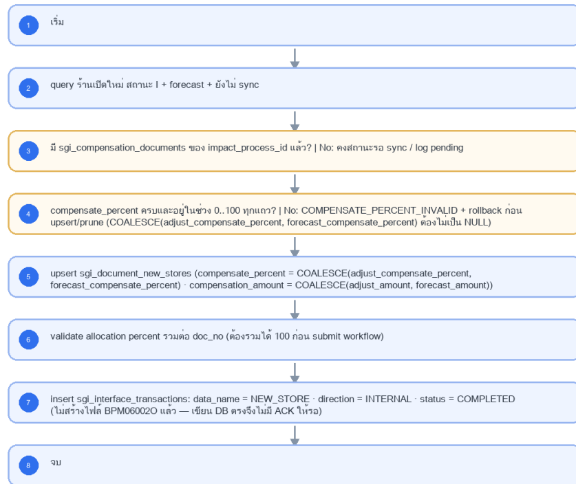
รูปที่ 1: Implementation flow: LLDD BE - Job 9 SyncNewStoreToDocument
