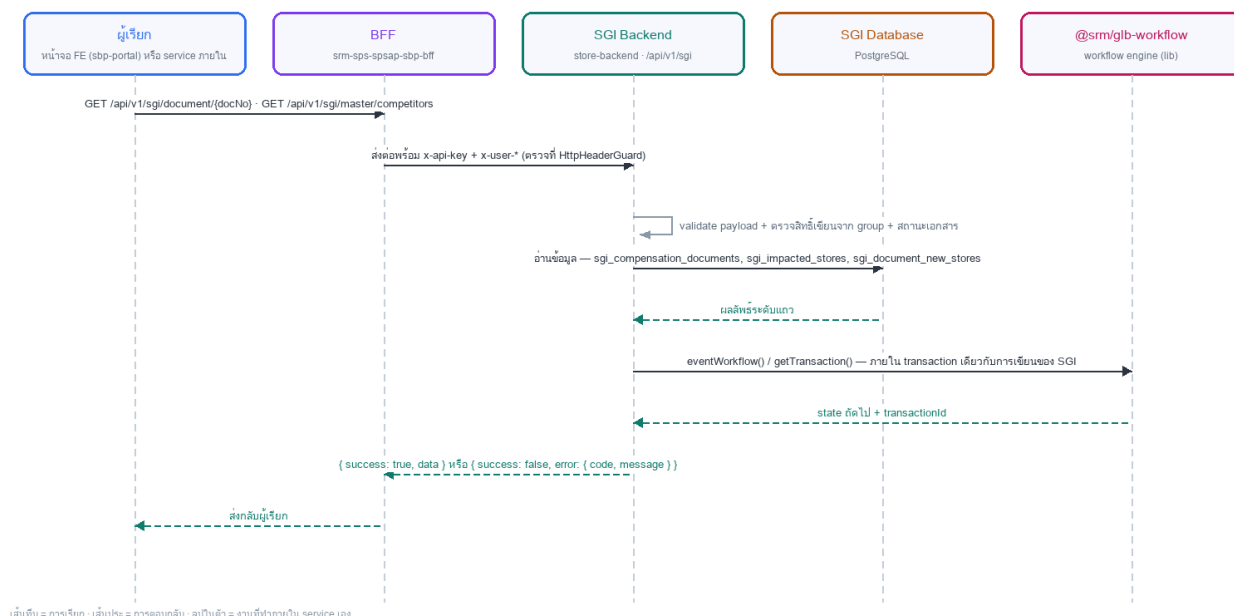
รูปที่ 2: Sequence diagram: LLDD BE - API Document Detail Aggregate
