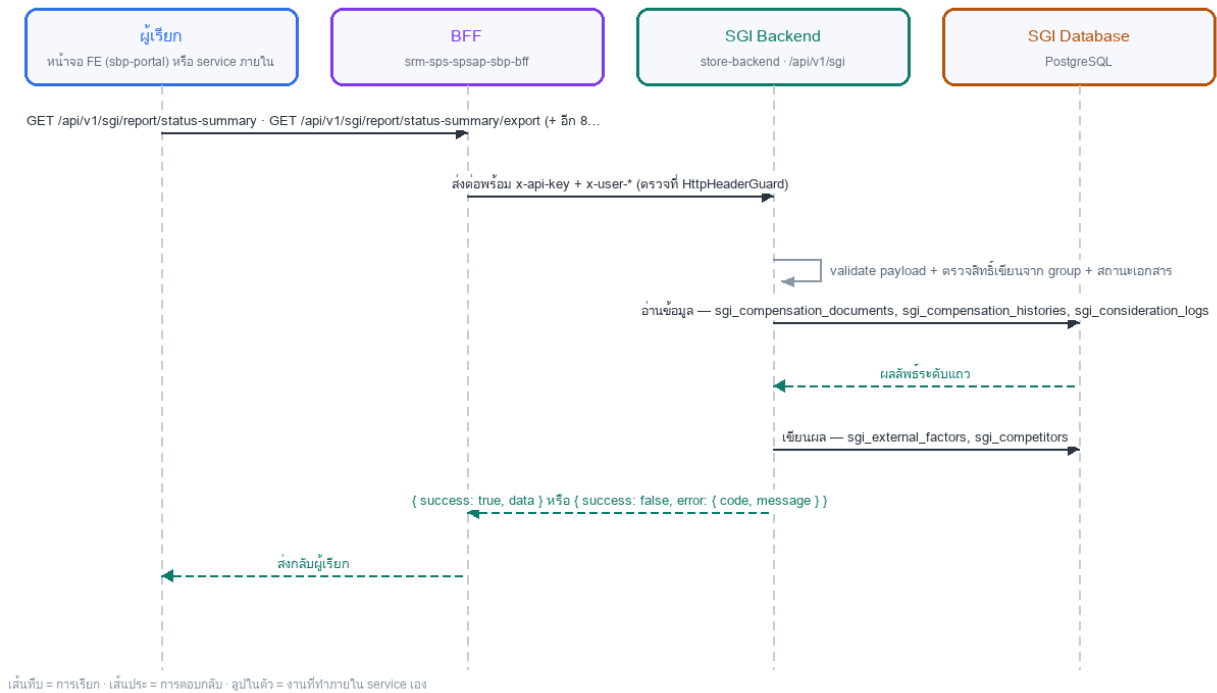
รูปที่ 2: Sequence diagram: LLDD BE - API Report and Master Data
