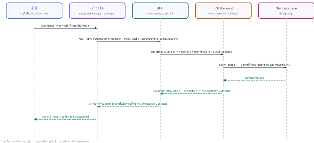
รูปที่ 2: Sequence diagram: LLDD FE - Document Detail Role 06 SBP DSA
