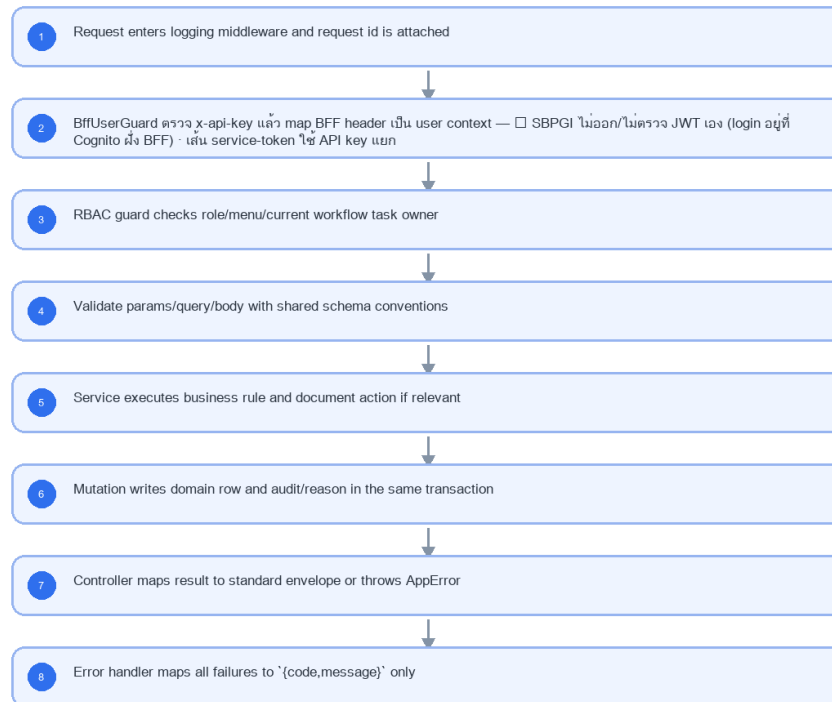
รูปที่ 1: Implementation flow reference: LLDD BE - API Common Contracts
