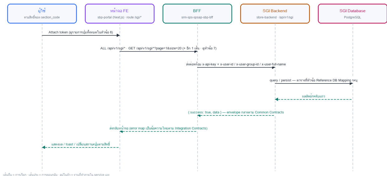
รูปที่ 2: Sequence diagram: LLDD FE - Integration Contracts
