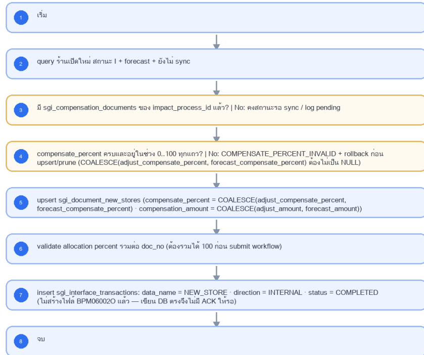
รูปที่ 1: Implementation flow: LLDD BE - Job 9 SyncNewStoreToDocument
