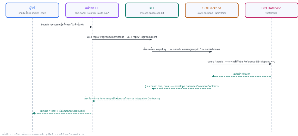
รูปที่ 5: Sequence diagram: LLDD FE - Document Lists
