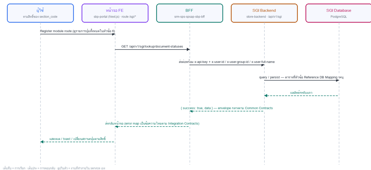
รูปที่ 2: Sequence diagram: LLDD FE - Application Foundation and Shared UI
