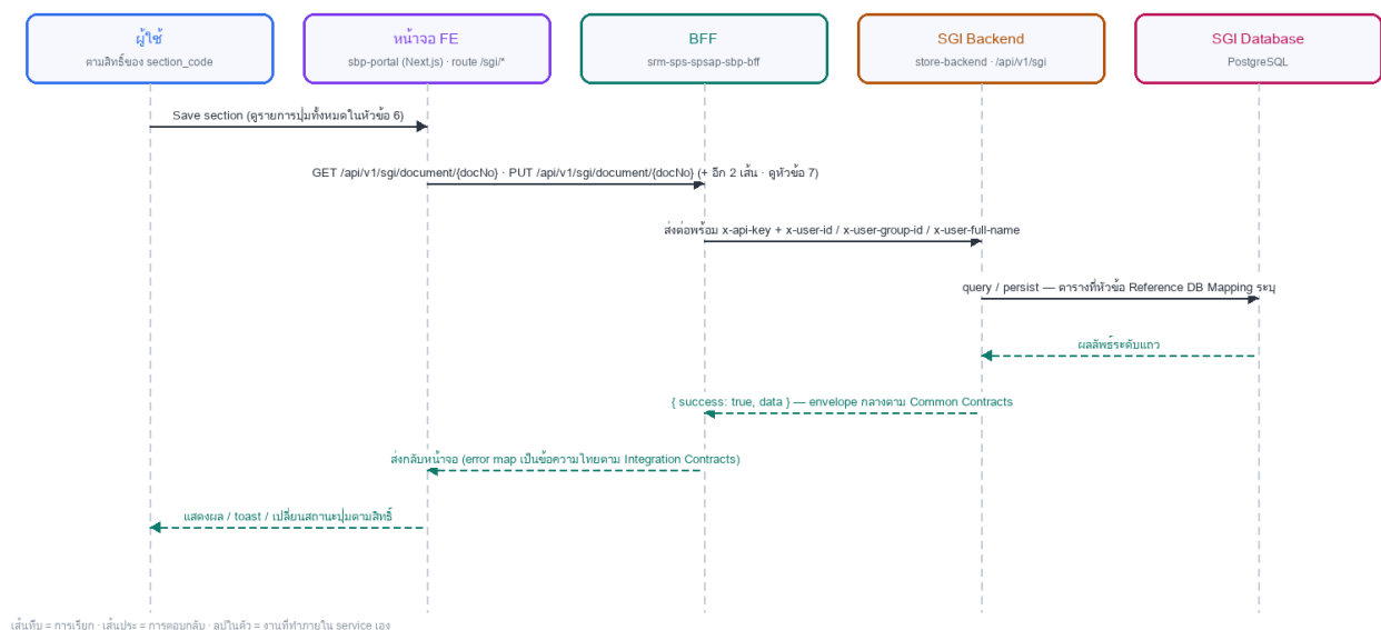
รูปที่ 5: Sequence diagram: LLDD FE - Document Detail and Action
