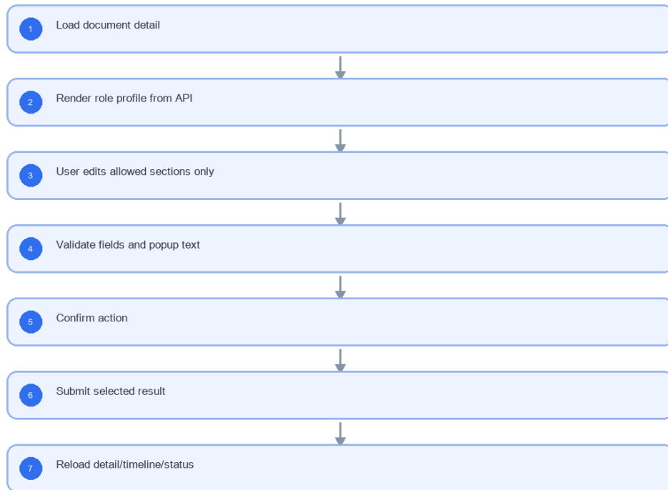
รูปที่ 4: Implementation flow reference: LLDD FE - Document Detail and Action
