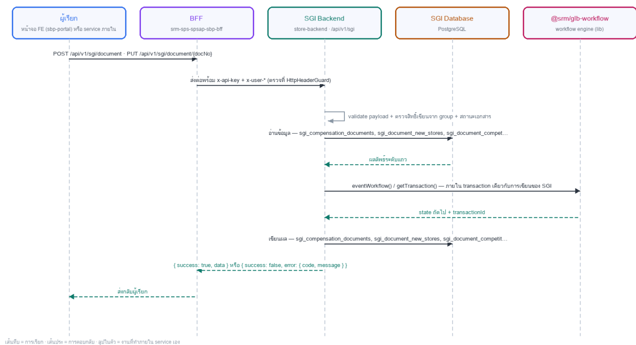
รูปที่ 2: Sequence diagram: LLDD BE - API Document Create and Update
