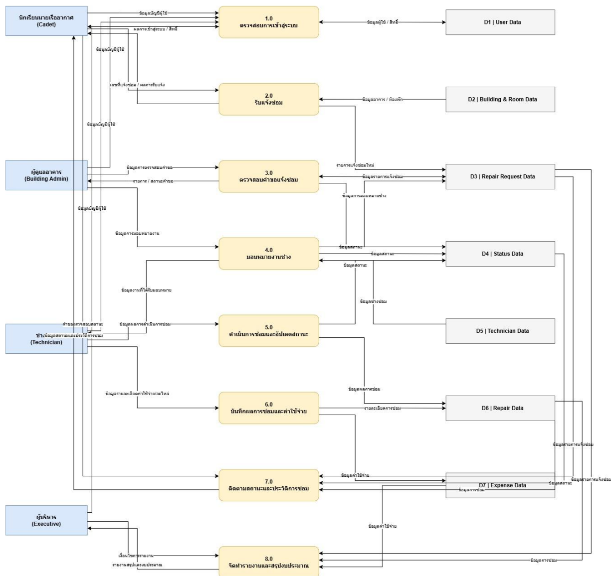
รูปภาพที่ 3 Data Flow Diagram Level-1
