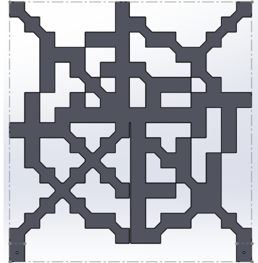
Pieza Simetrica, plegar 90º según lado Der/Izq
