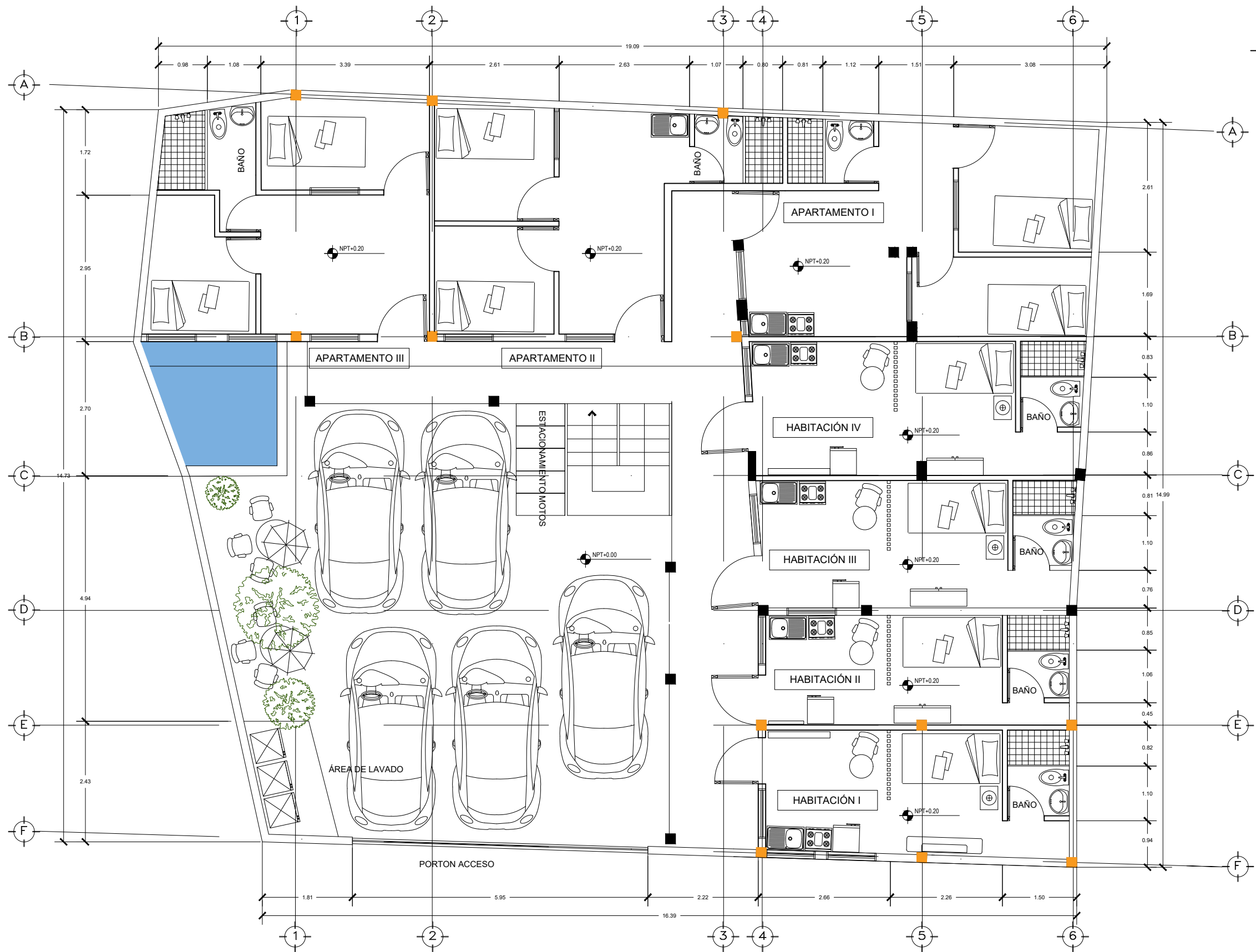
PLANTA ARQUITECTÓNICA NIVEL 1
