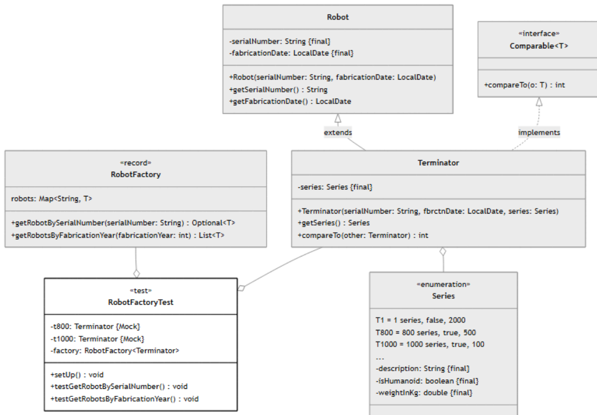
Abbildung 2: Klassendiagramm Aufgabe 2
